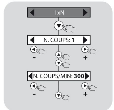
MODE 1xN
